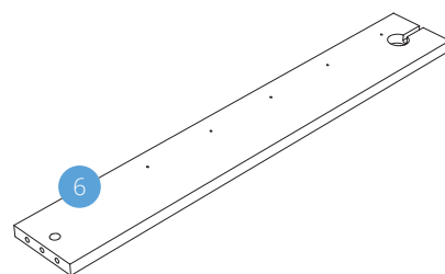
Царга левая передняя 1 шт.
